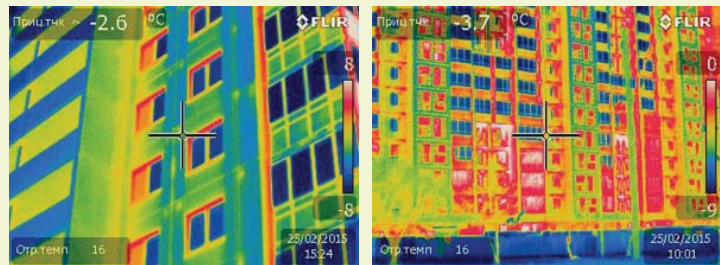
Тепловизионная съемка многоквартирного дома
