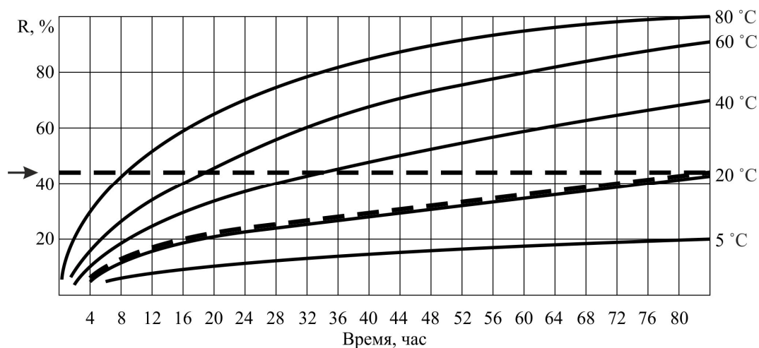
Рисунок К.3. Температурный график
