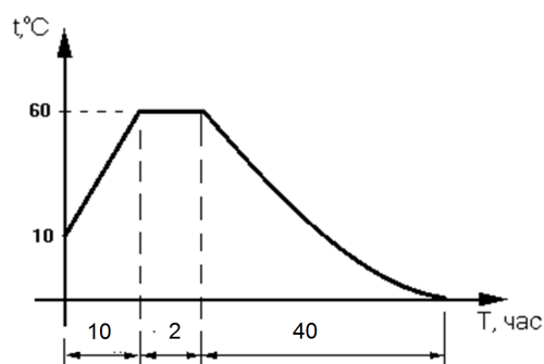
Рисунок К.1 – Температурный режим твердения бетона
