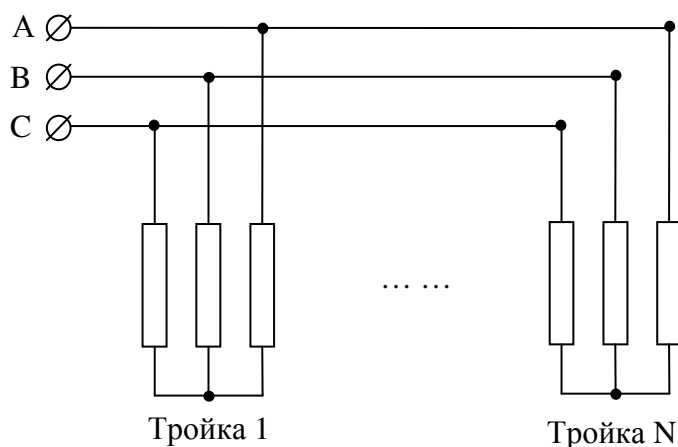
Рисунок 7.1 – Схема соединения проводов звездой
