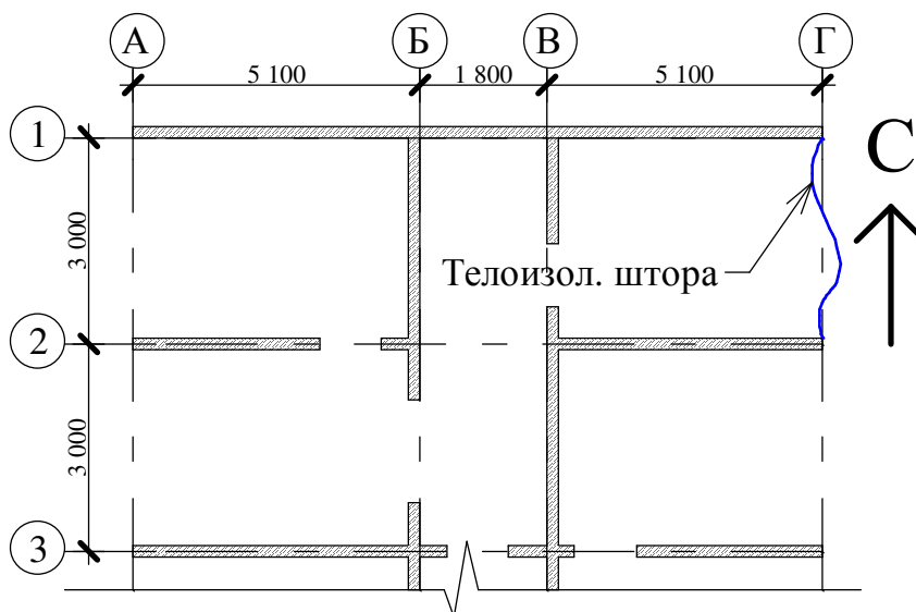
Рисунок Е.1 – Схема расположения монолитных конструкций
