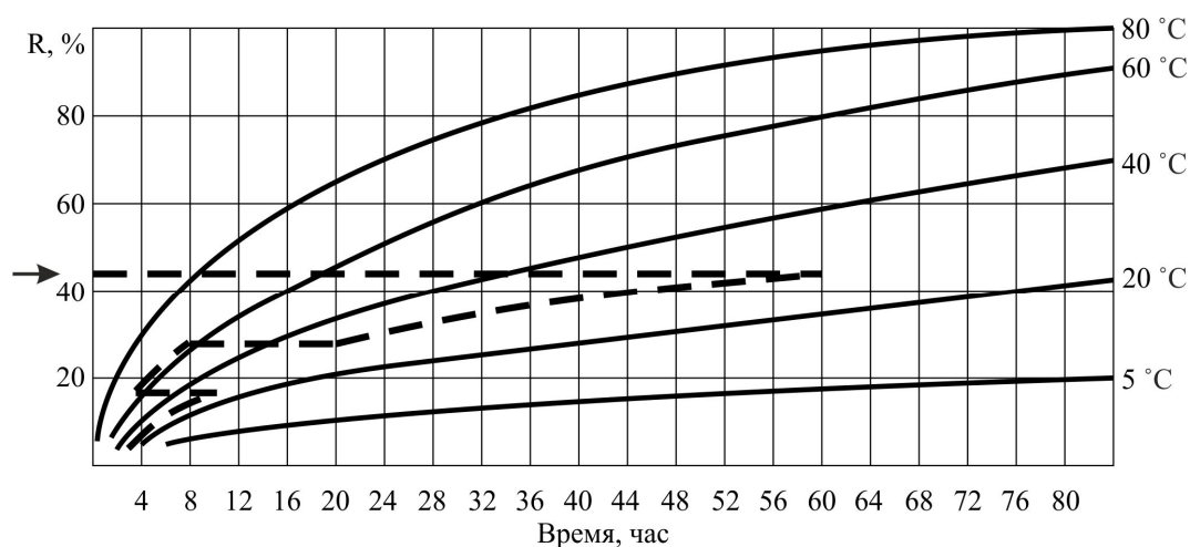
Рисунок К.2. Температурный график
