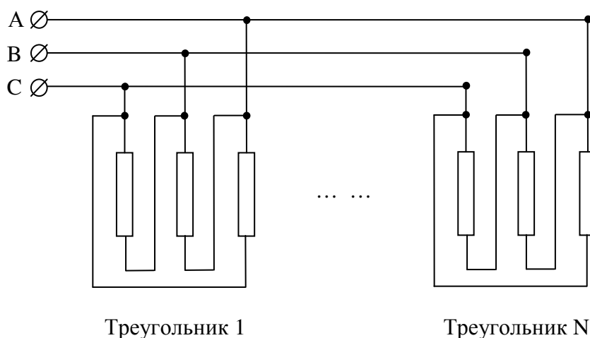
Рисунок 7.2 – Схема соединения проводов треугольником
